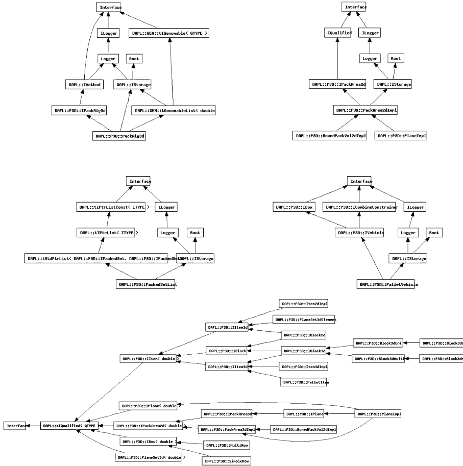
Рис. 6. Локальная иерархия базовых классов алгоритма.
