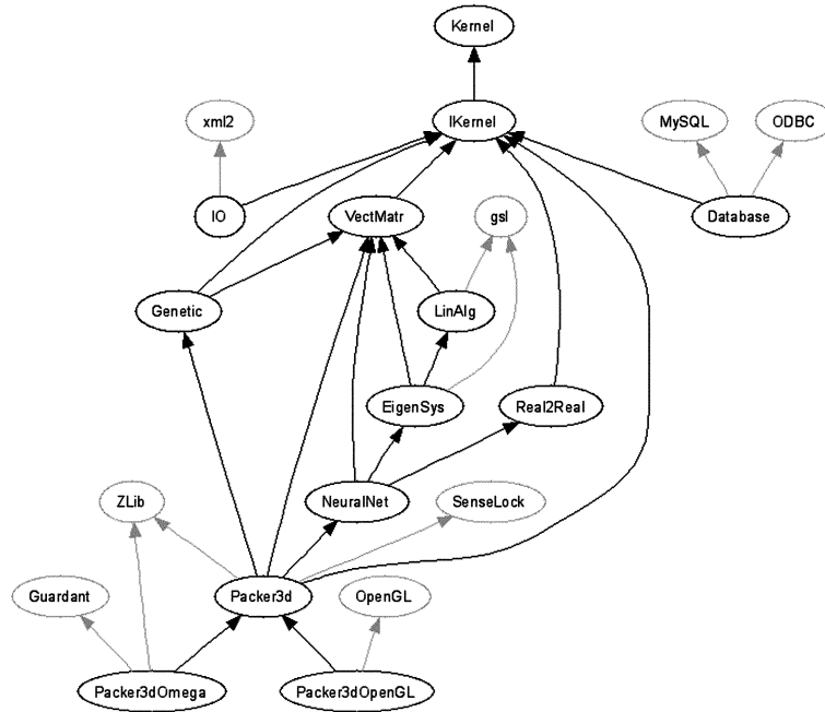
Рис. 4. Зависимость библиотек C++ классов.
