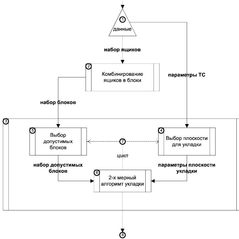
Рис. 1. Схема алгоритма.
